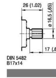
S4 DIN 5482 B17x14 Coppia Max Max Torque 130 Nm
