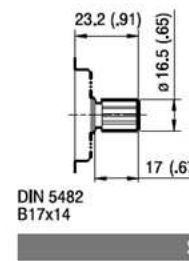
S3 DIN 5482 B17x14 Coppia Max Max Torque 130 Nm
