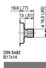
S0 DIN 5482 B17x14 Coppia Max Max Torque 130 Nm
